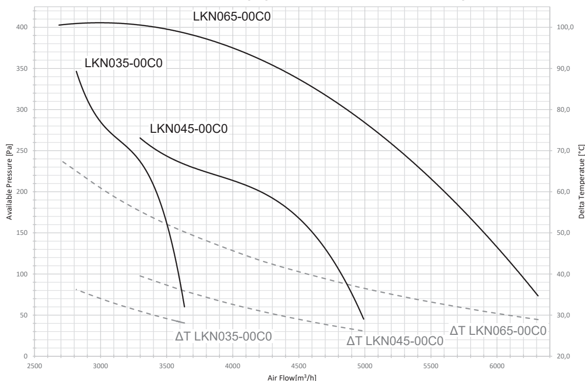
Schema "luchtdebiet - drukverlies - verhoging luchttemperatuur" van de centrifugale verhitters LKN
